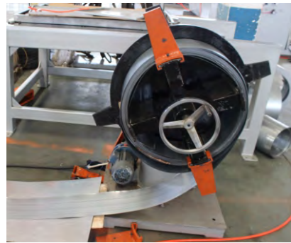
开料架 / Pay-off
